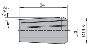
Цанга зажимная тип 407E для хвостовиков диаметром 6-12,7 мм
