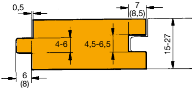
Profile 3: AF 200 2
